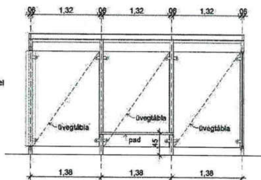
ELÖLNÉZET
