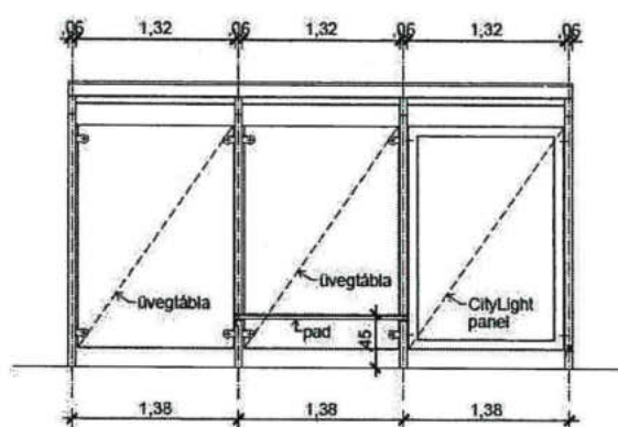
ELŐLNÉZET
