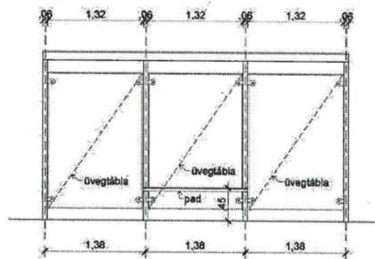
ELÖLNÉZET
